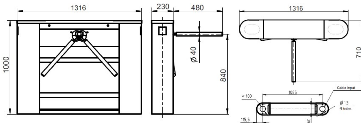
Medidas GALAXY-ACR
